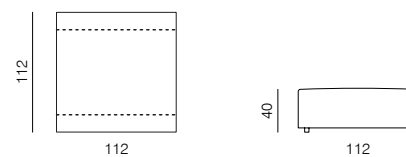
POUF 112 dimensions 112 × 112 × 40 cm
